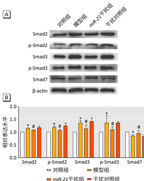
图 4 BeSO 4 处理 A549 细胞 48 h 后 Smad 蛋白相对表达水平 Figure 4 Relative expression levels of Smad in A549 cells treated with BeSO 4 for 48 h
